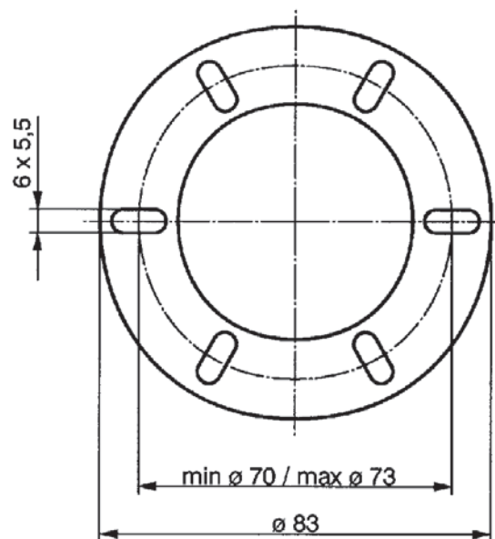
Befestigungsflansch Mounting flange
