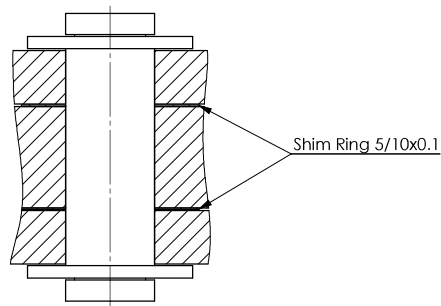
B-B (5 : 1)
