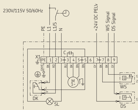
Schaltbild 4
