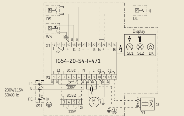
Schaltbild 7
