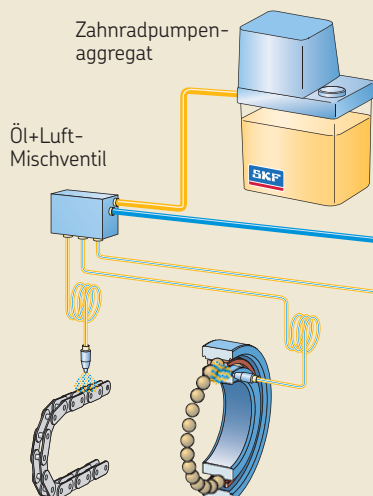
Öl+Luft-System
