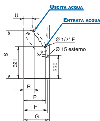
DIMENSIONI (mm)
