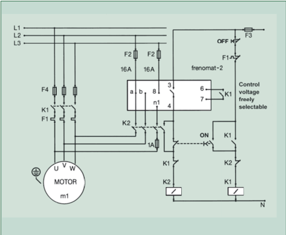
Circuit diagram ►
