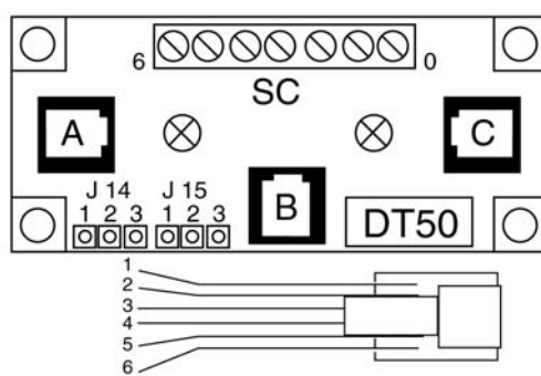
RJ12 Pinbelegung
