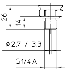
G1/4A DIN EN ISO 1179-2 (DIN 3852-11) model E
