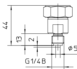
G1/4B DIN EN 837-1
