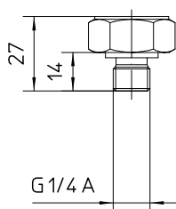
G1/4A DIN EN ISO 1179-2 (DIN 3852-11) model E
