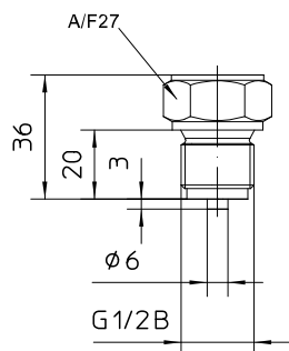
standard G1/2B DIN EN 837-1
